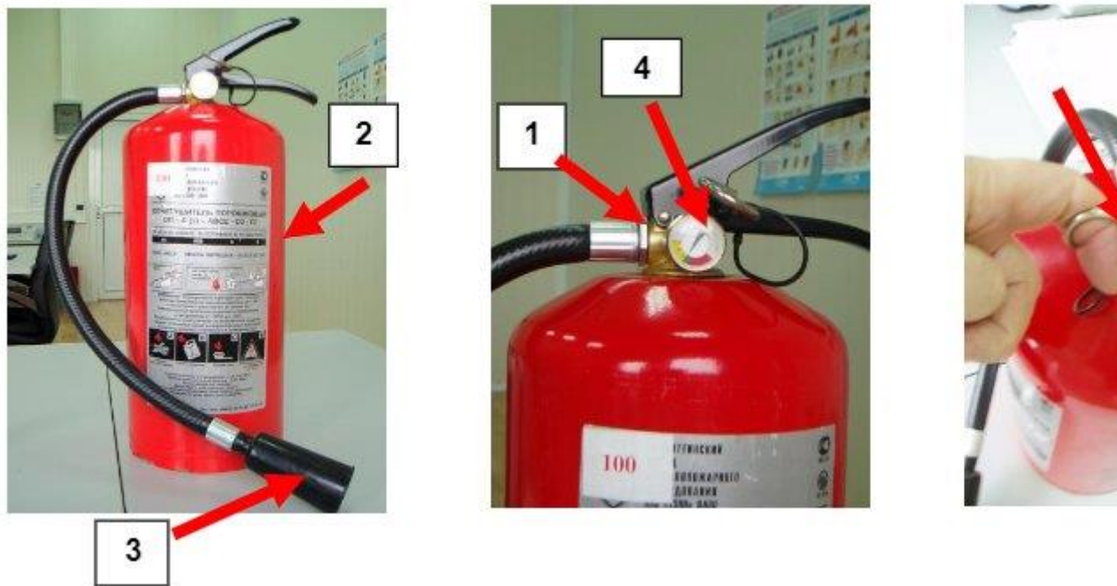
Рис.1. Порошковый огнетушитель типа ОП-4(з)
